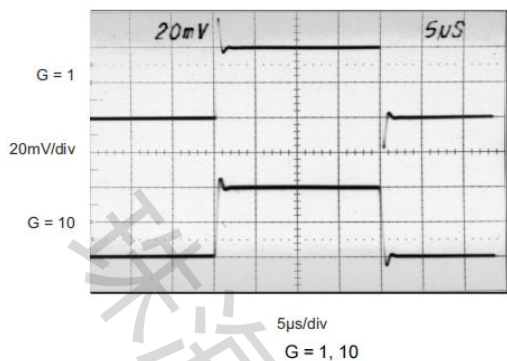
图 19. Small Signal
