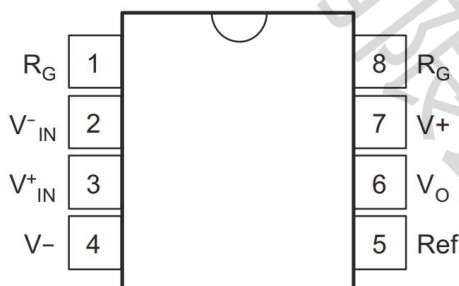
芯片引脚描述
