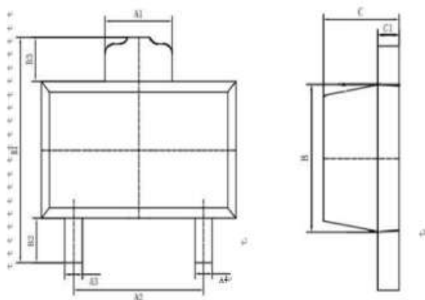
SOT-89-2L
