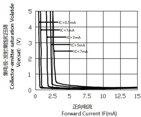
集电极-发射极饱和电压与正向电流特性曲线 Collect-emitter Saturation Voltage vs. Forward Current
