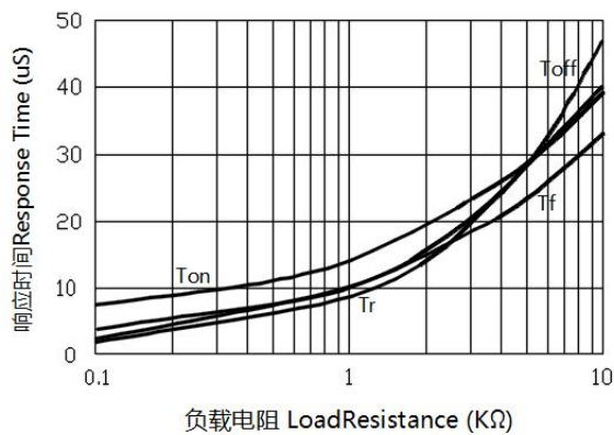
响应时间与负载电阻特性曲线 Response Time vs. LoadResistance
