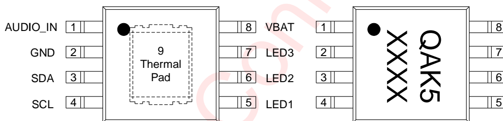
AW2028HSPR (Top View)
