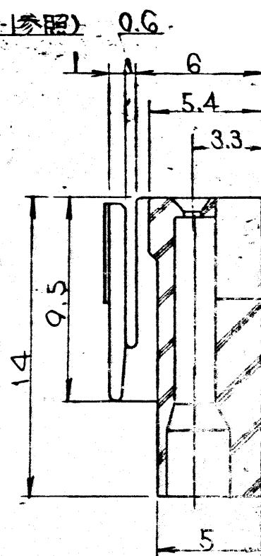
A-A 斷面圖
