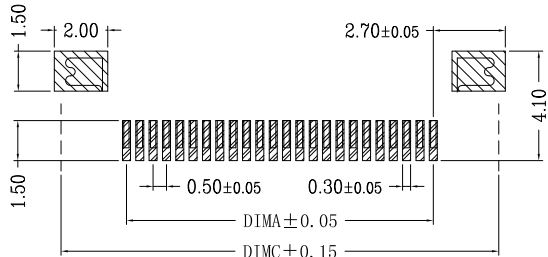
适用线路板
