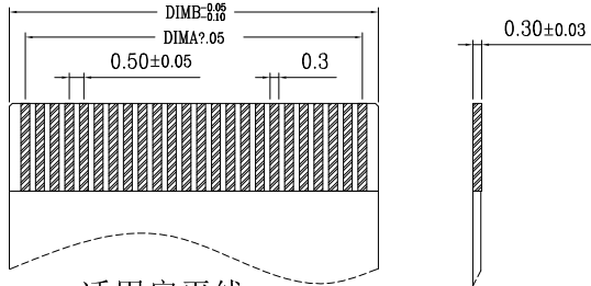
适用扁平线
