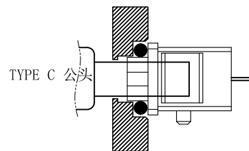
组装示意图
