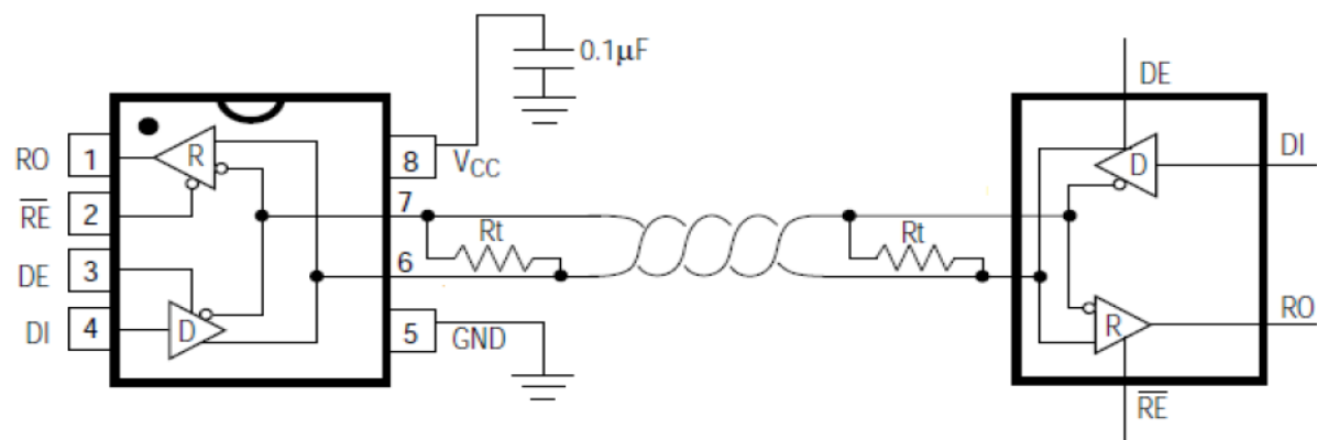
图 1: MAX1487EESA-TD典型半双工应用电路
