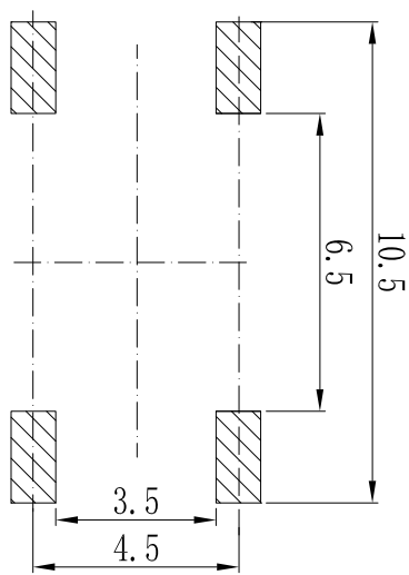
PCB线路板安装图(±0.1)
