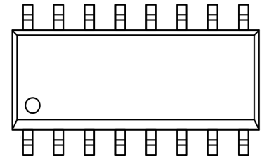
SOP16
