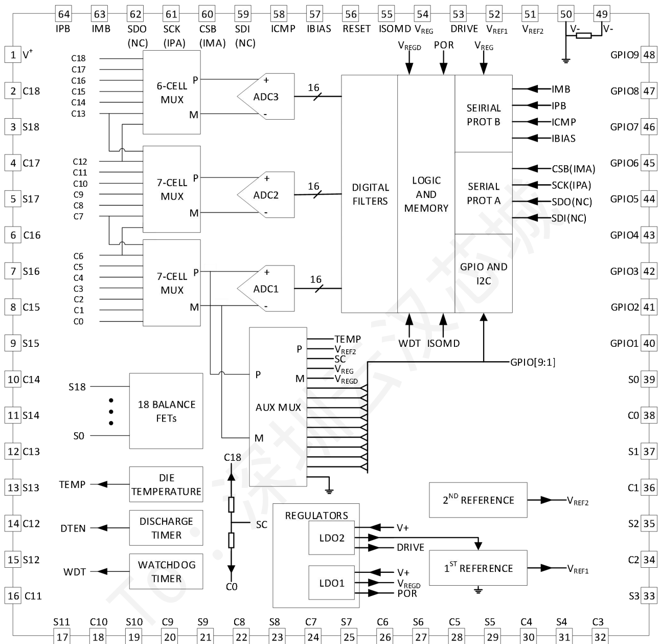
图 1-1 系统框图
