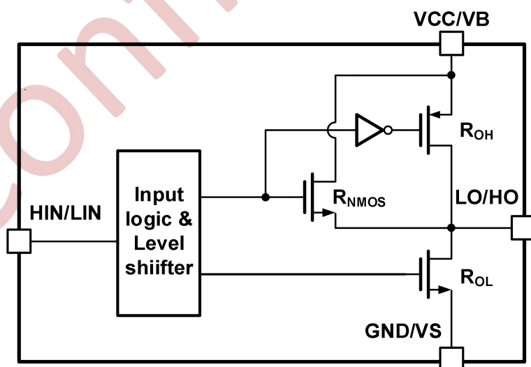
图 10-2 NSG6025 输出级示意图
