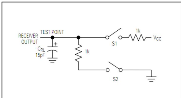
图 9 接收器使能/禁能时序测试电路
