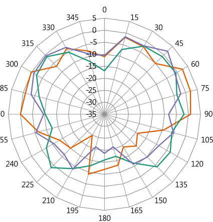
YZ-Plane Gain
