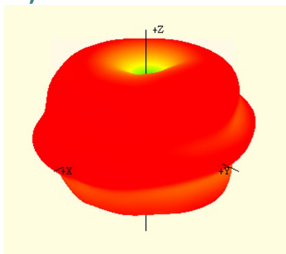
6525 MHz
