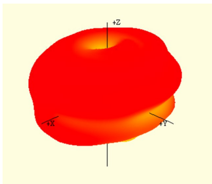
7125 MHz
