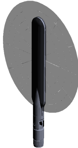
YZ-Plane Gain
