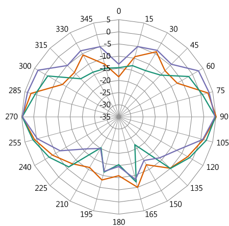
5150 MHz
