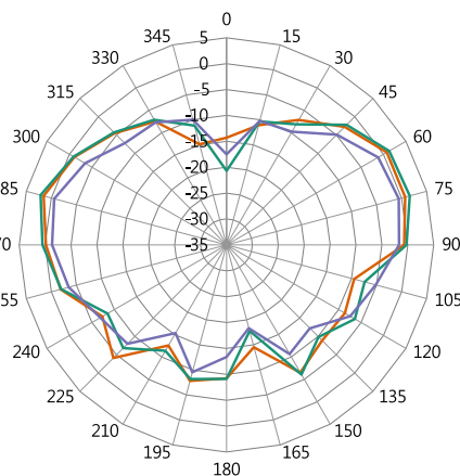
2450 MHz
