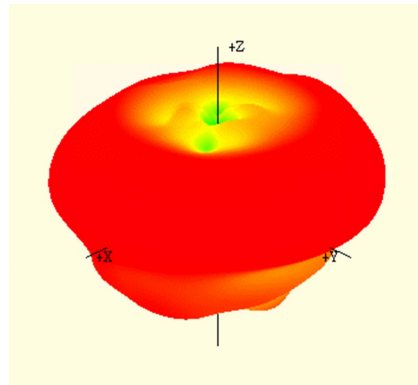
2450 MHz
