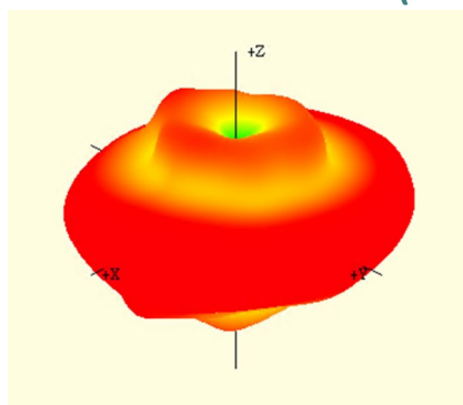
5150 MHz
