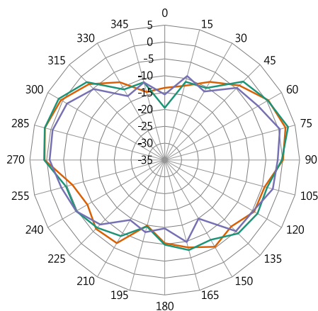
2400 MHz
