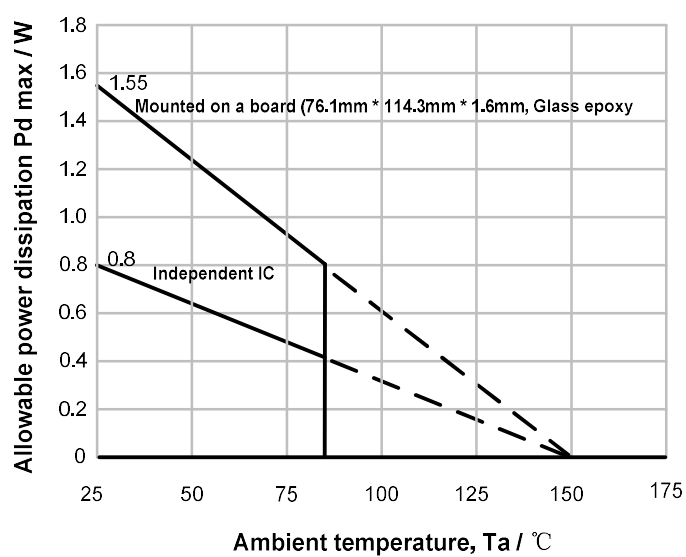
图 2 HTSSOP28 with PAD 额定参数曲线图
