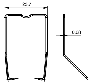
18FF-H5 (金属卡簧)
