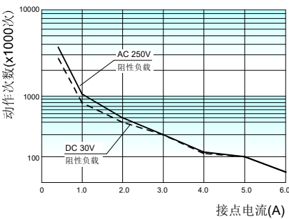
阻性电耐久性曲线 (4Z)
