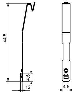
18FF-H5 (金属卡簧)
