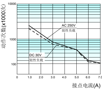
阻性电耐久性曲线 (2Z)
