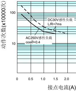
感性电耐久性曲线 (4Z)
