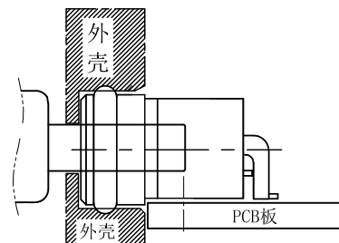
组装示意图
