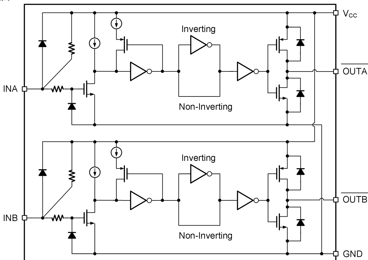
IX4426NTR功能框图
