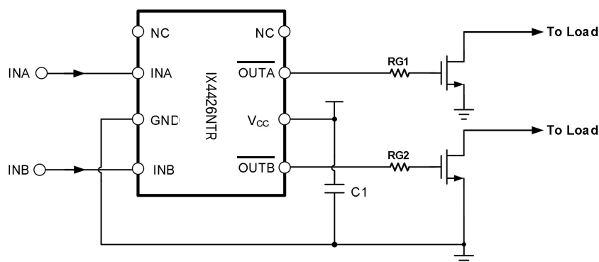
IX4426NTR 反相典型应用电路图
