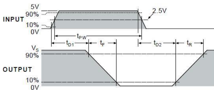
输入输出(反相)波形图
