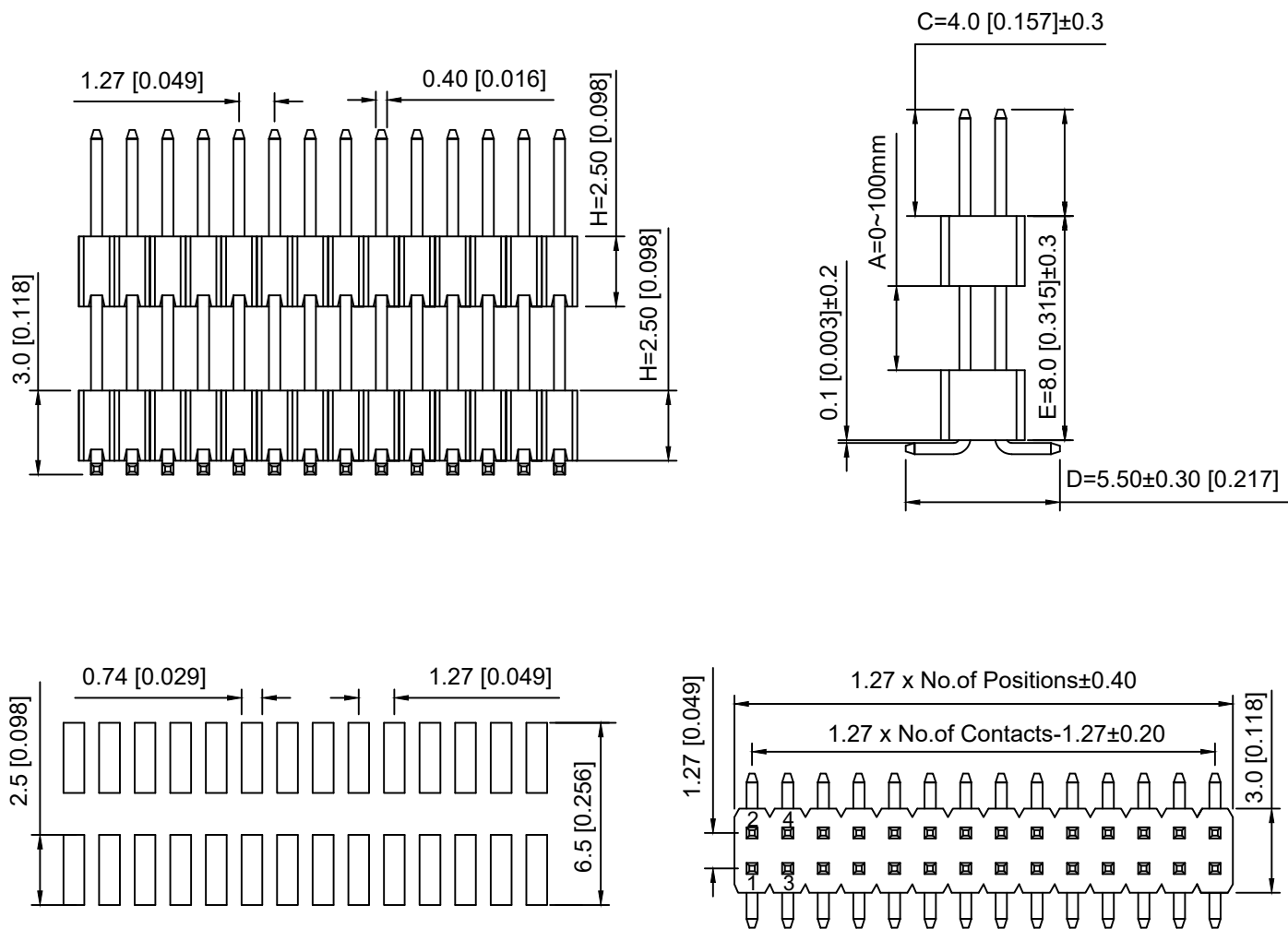
P.C.B LAYOUT
