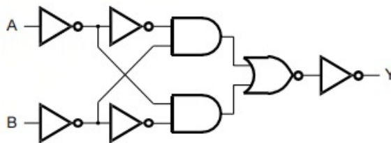
图 3 逻辑框图
