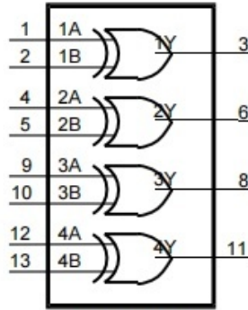
图 1 逻辑符号
