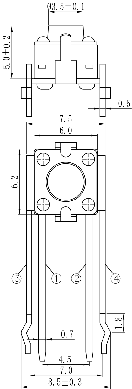
PCB线路板安装图(±0.1)
