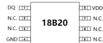
MSOP8 (18B20U)
