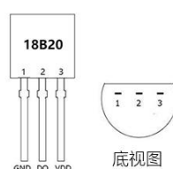
TO-92 (18B20)
