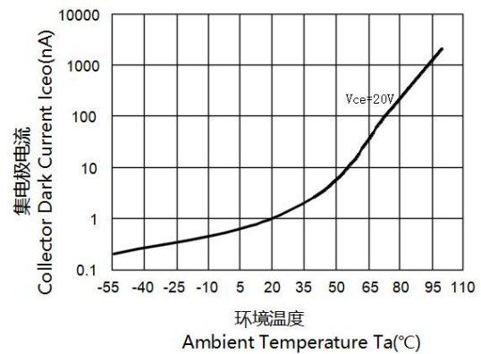
集电极暗电流与环境温度特性曲线 Collector Dark Current vs. Ambient Temperature
