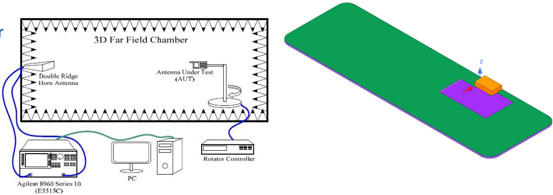
Fig.2 暗室示意图 FAR-field Chamber
