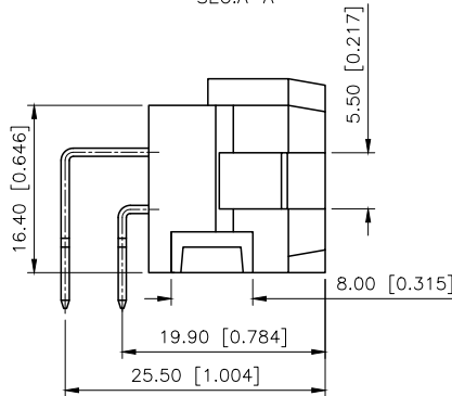
SEC:A-A
