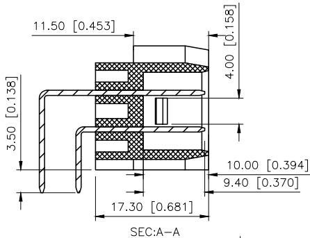
SEC:A-A
