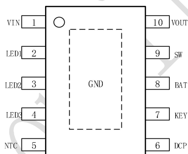
ESOP10
