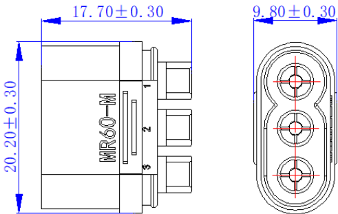
带后盖堆叠尺寸
