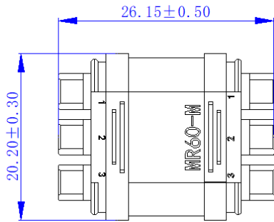
带后盖互配尺寸
