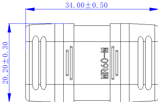
带后盖互配尺寸
