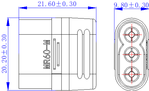
互配尺寸
