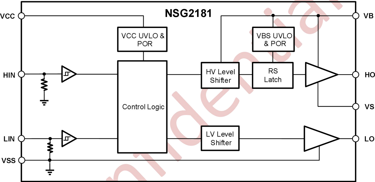
图 10-4 NSG2181 功能框图
