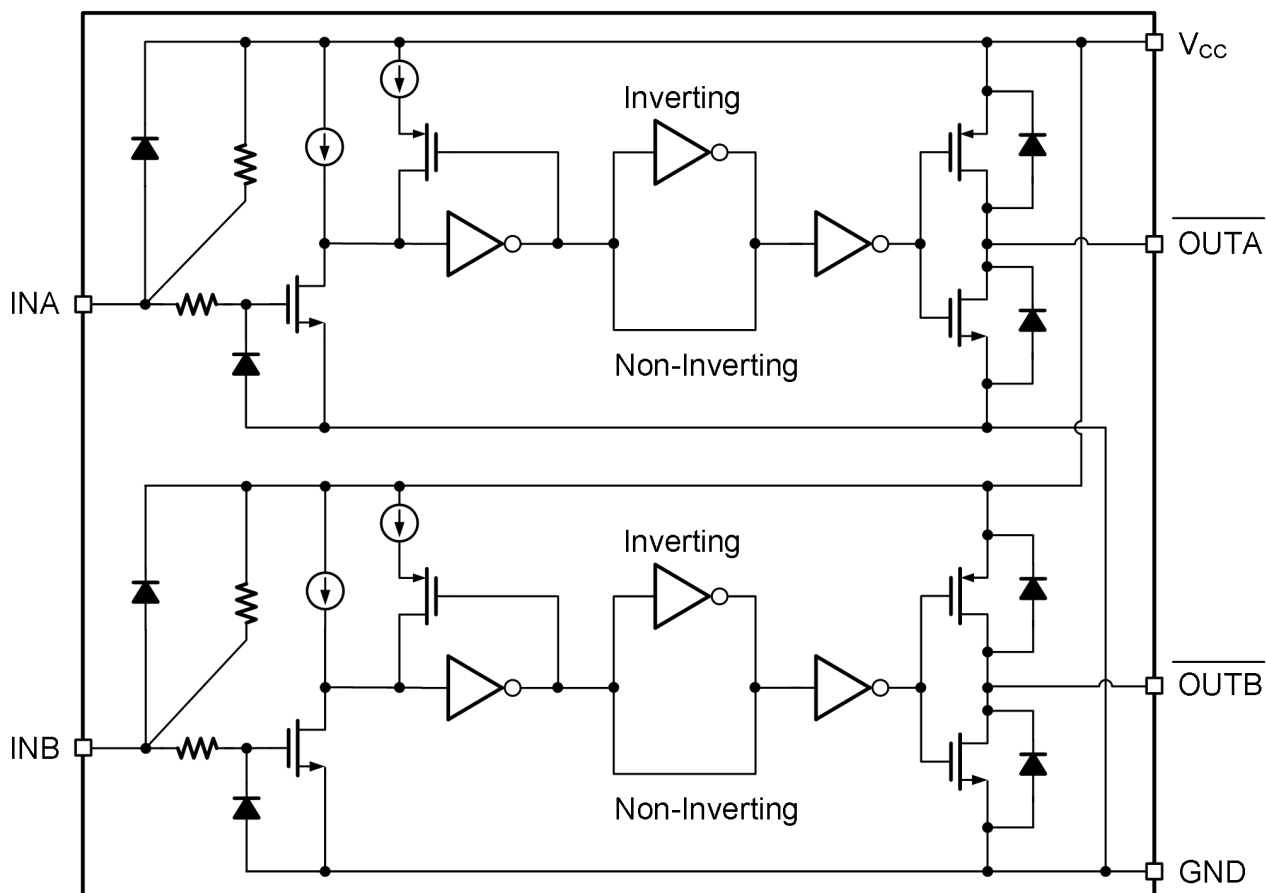
IR4426STR功能框图
