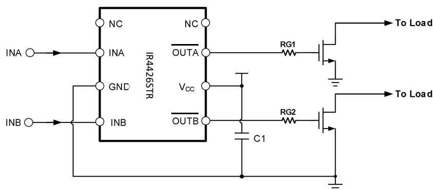
IR4426STR反相典型应用电路图
