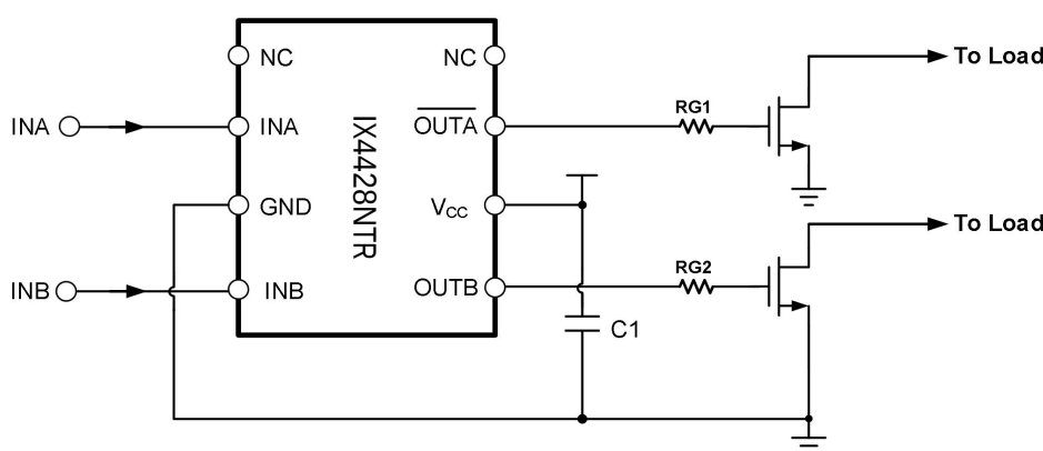
IX4428NTR典型应用电路图
