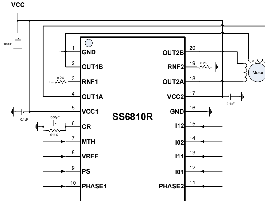
图 2. 应用原理图
