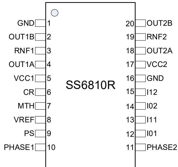
图 3. 顶视图
