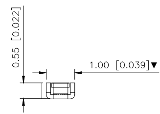
SECTION D-D
