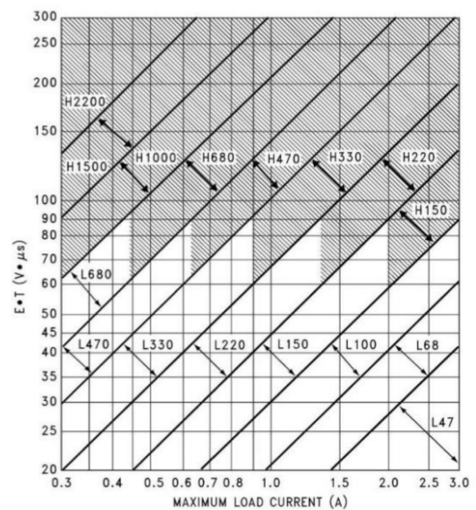
LM2576HV-ADJ
