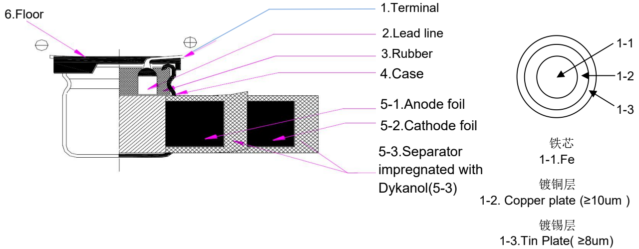
电容器 Capacitor
