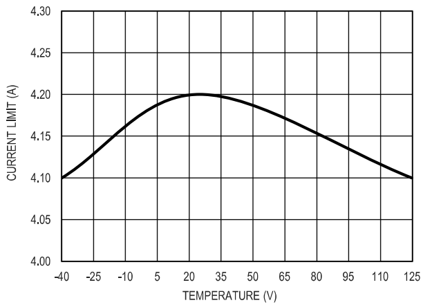
图 17. 输出限流值和温度的关系
