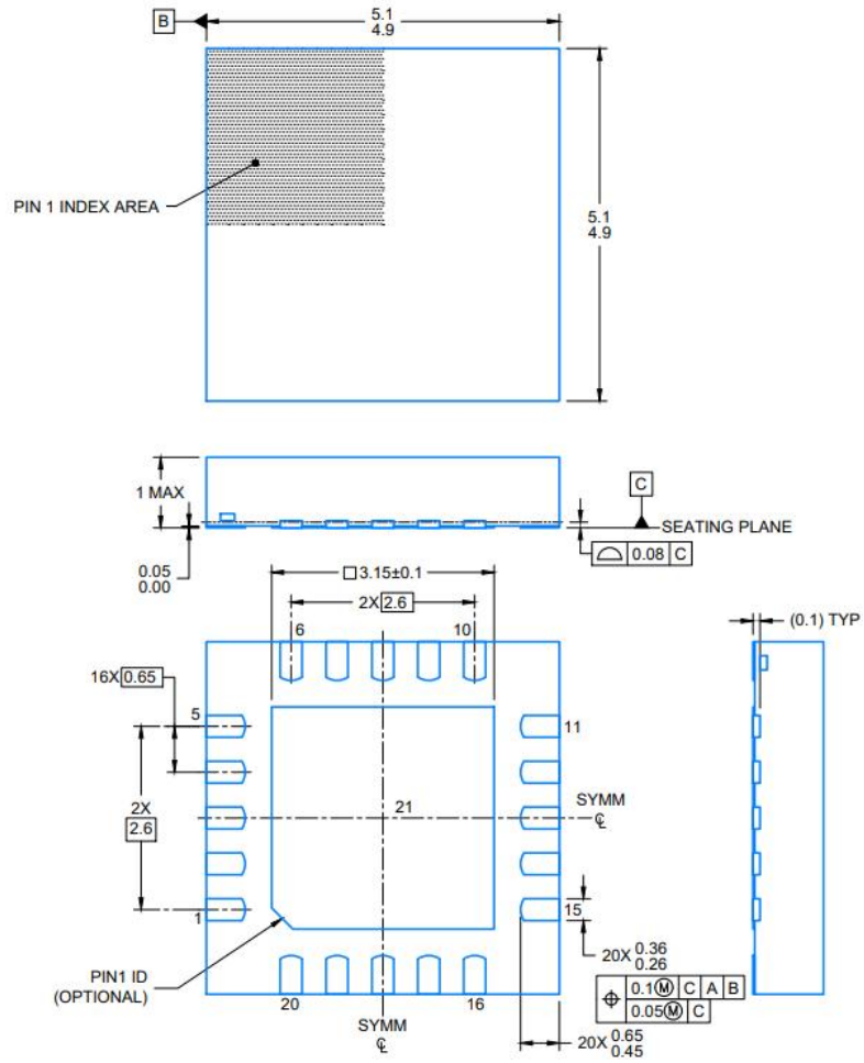
图 36.20 引脚 QFN (5 毫米 x 5 毫米) 所有线性尺寸均以毫米为单位
