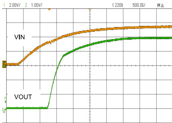
图 23. 软启动, V_{IN} = 5.3V , V_{OUT} = 5.0V , I_O = 3A
