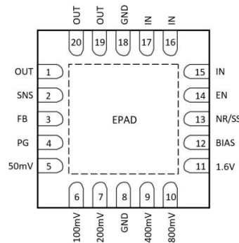
QFN 20-LEAD (3.5mm×3.5mm) 裸露焊盘必须焊接到 PCB 上
