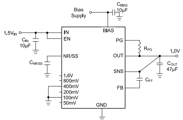
图 29 无需外部电阻的输出电压设置
