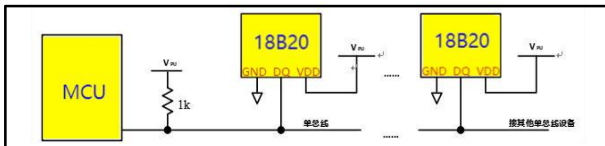
图 9.1 外部供电模式示意图
