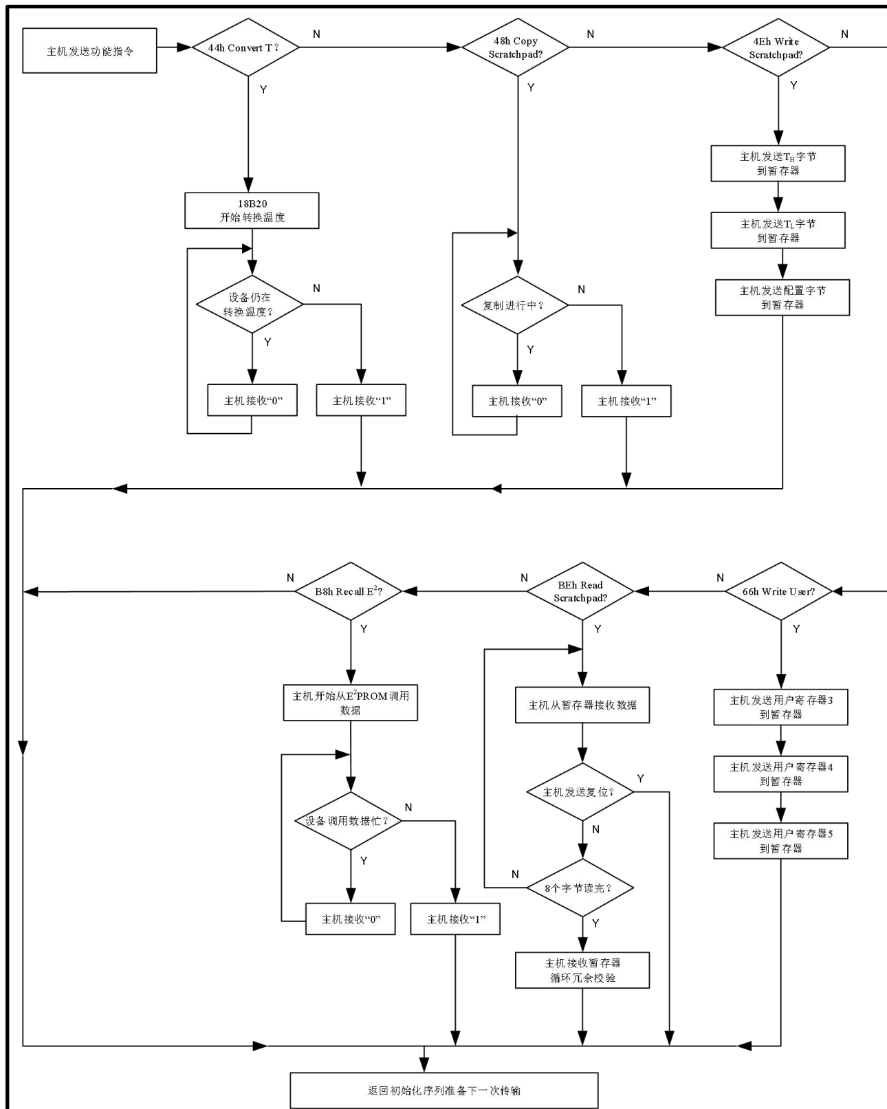
图 11.5-2 功能指令流程图
