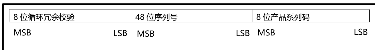
图 10.1 64 位 ROM 编码
