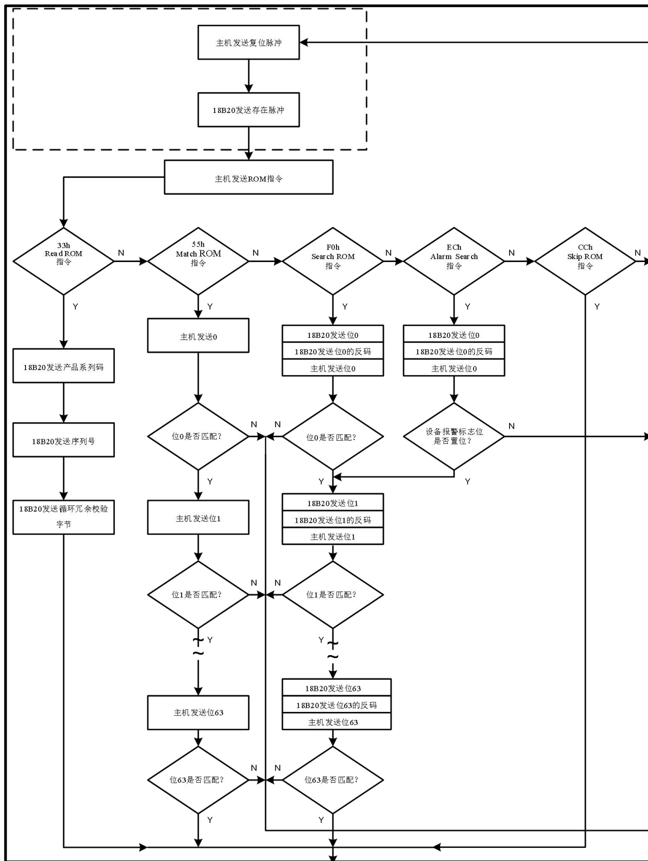
图 11.5-1 ROM 指令流程图
