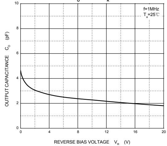
C_O - V_R
