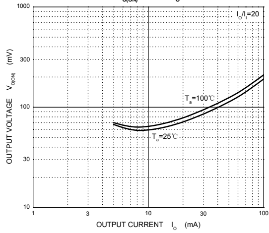
V_{OL(ON)} - I_O
