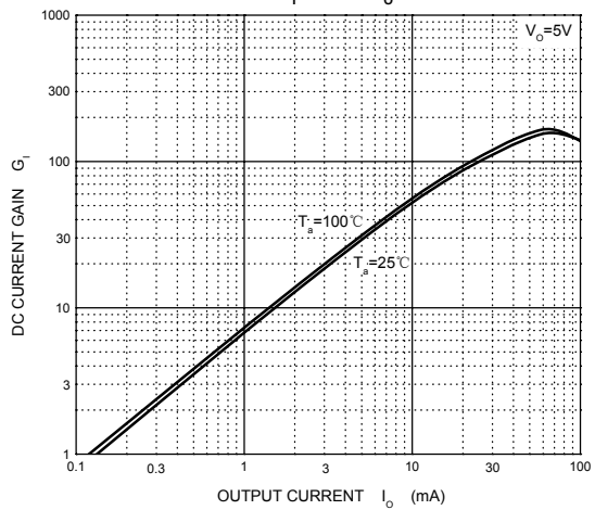
G_I - I_O
