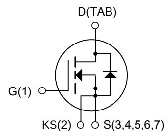
TO-263-7L (TO-263-7-13)
