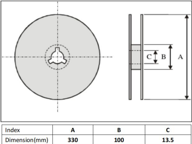
Reel dimensions
