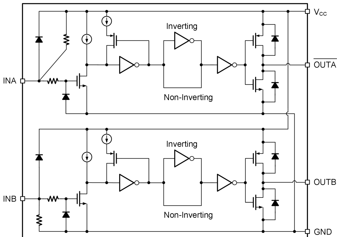
IR4428STRPBF 功能框图
