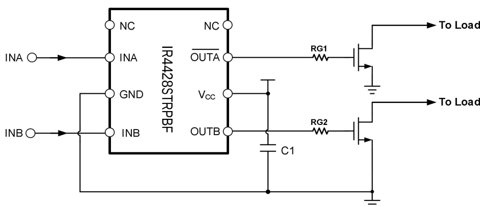
IR4428STRPBF典型应用电路图
