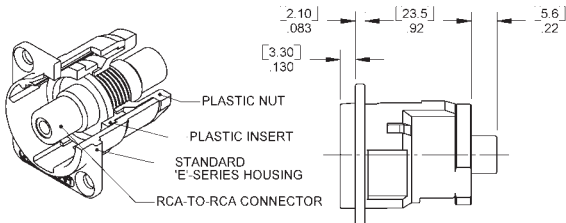
EHRCA2
