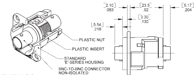
EHBNC2
