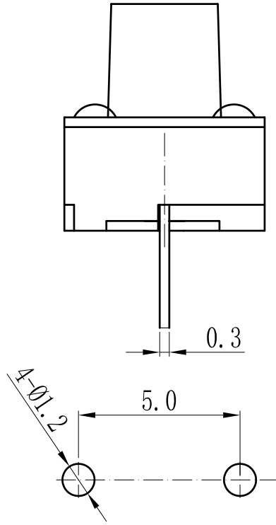
PCB线路板安装图(±0.1)
