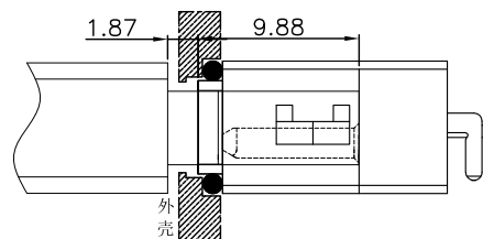
组装示意图
