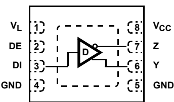
ISL3296E, ISL3297E, ISL3298E (8 LD TDFN) TOP VIEW
