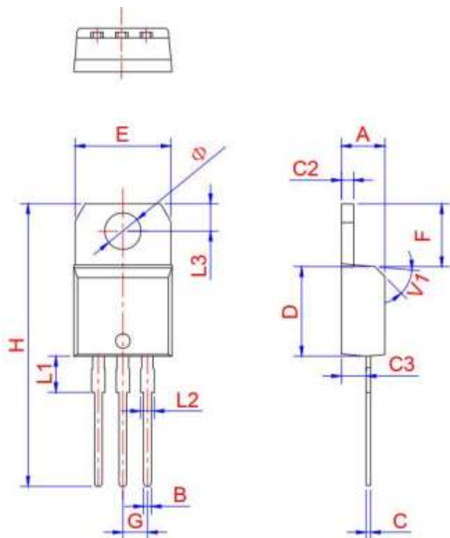
TO-220A Ins
