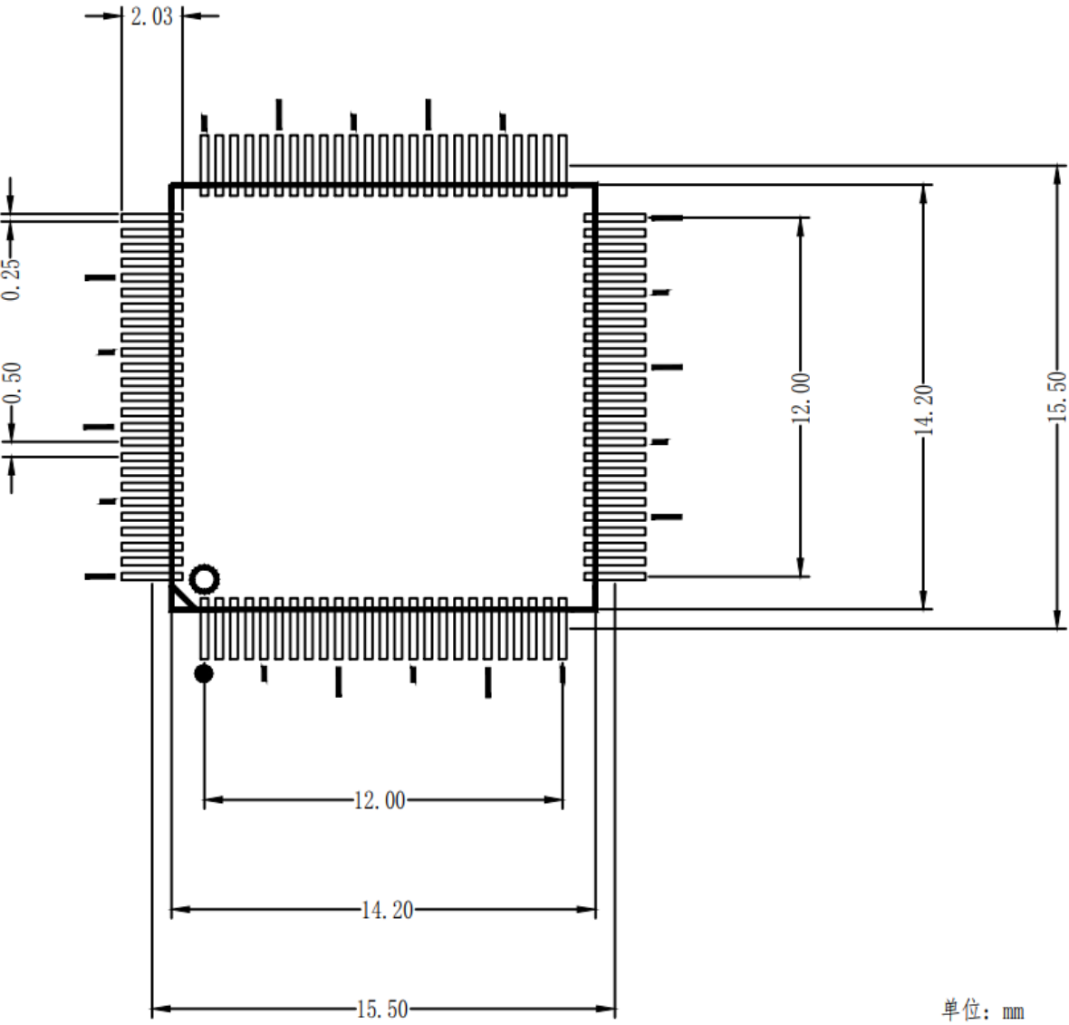
图 8 CQFP100 封装推荐焊盘图
