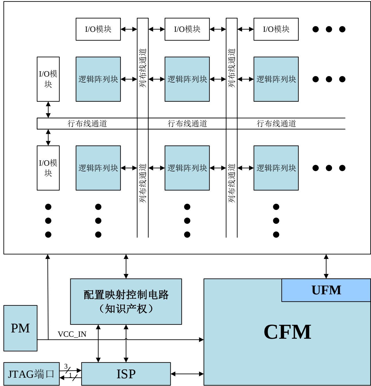
图 1 功能框图
