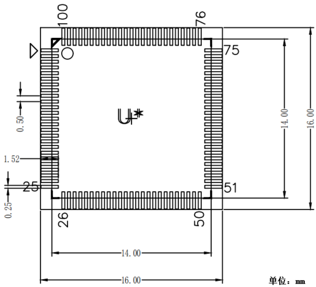
图 7 PQFP100 封装推荐焊盘图
