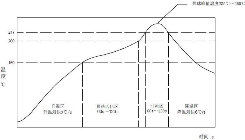
图 11 无铅回流曲线
