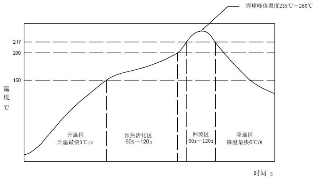
图 14 无铅回流曲线
