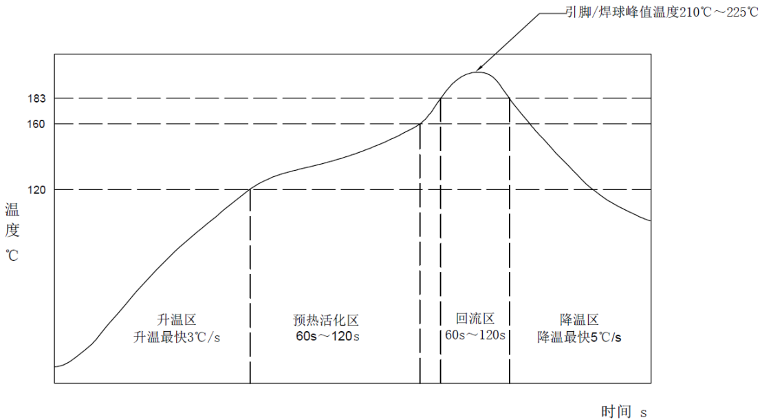
图 13 有铅焊料 Sn63Pb37 回流曲线
