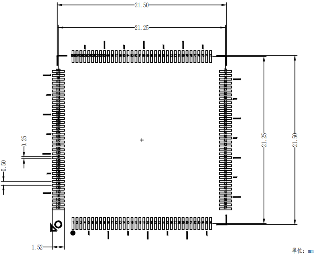
图 9 CQFP144 封装推荐焊盘图
