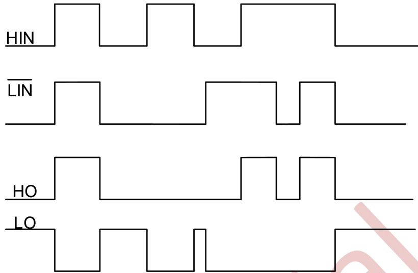
图 9-1 NSG2023 输入输出时序波形
