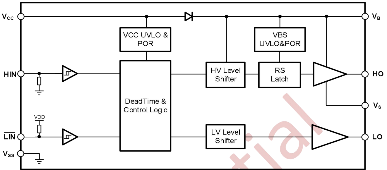
图 10-1 NSG2023 功能框图
