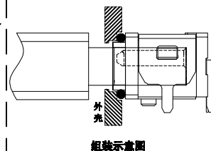
组装示意图
