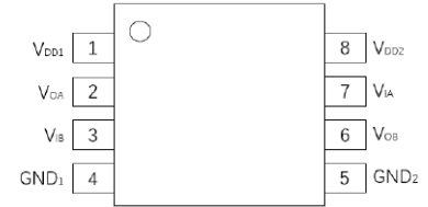
图 2. 管脚定义
