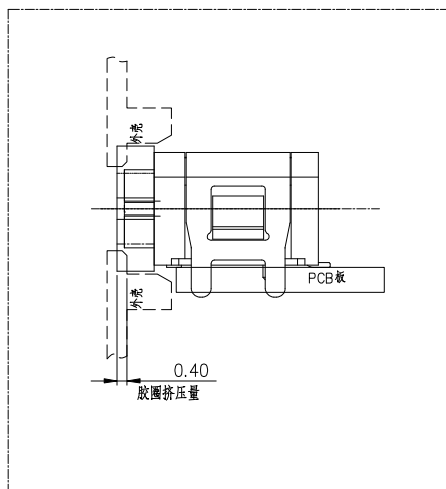
组装示意图
